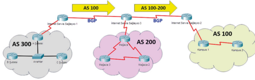
Görsel 5.89: BGP ve yol vektörü protokolü kullanımı
