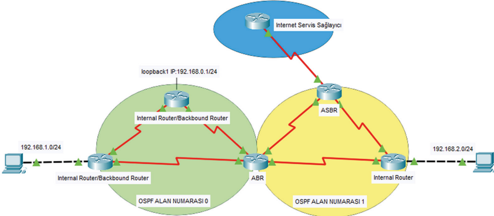
Görsel 5.30: OSPF yönlendirici çeşitleri
