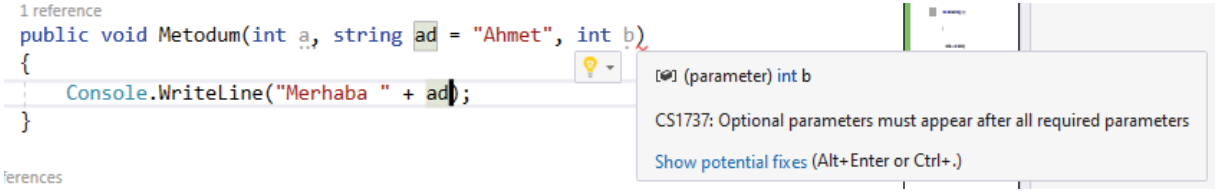
Görsel 3.7: Varsayılan parametrelerin hatalı kullanımı
