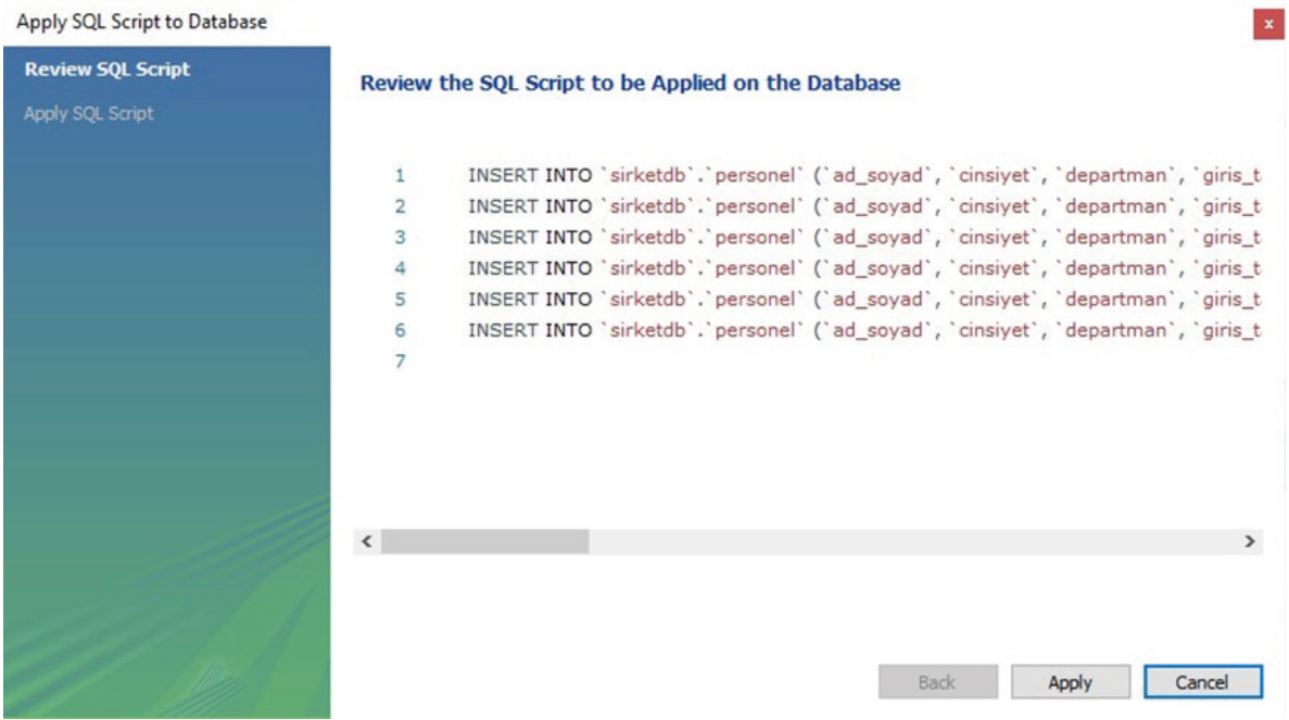
Görsel 6.40: Personel tablosu veri girişi SQL komutları
