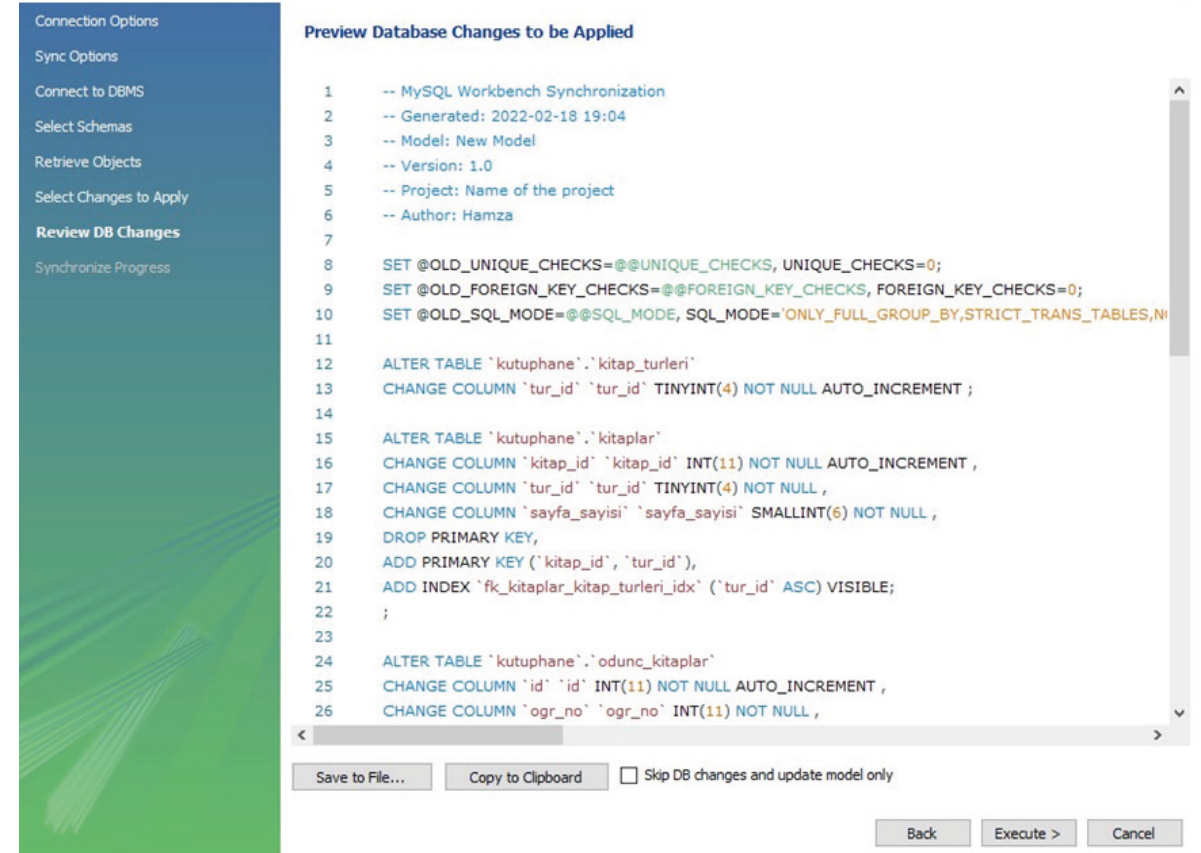
Görsel 6.80: İlişkiyi oluşturacak olan SQL komutları
